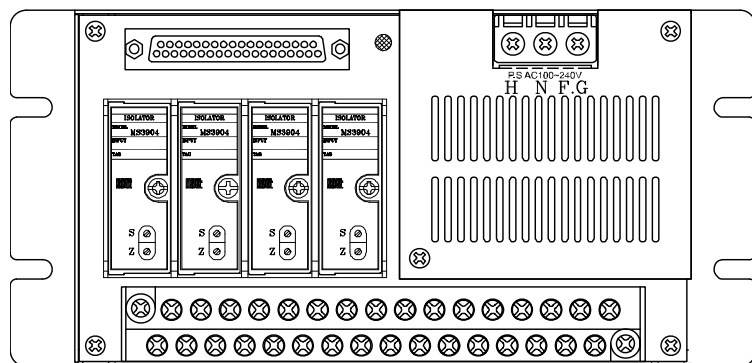
正面図
